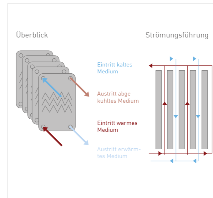
Abb. 7: Prinzip eines Plattenwärmeübertragers
