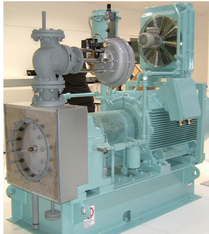
Abb. 5: Einstufige Kompakt-Dampfturbine (SST-040 von Siemens, für trockenen Sattdampf bis 400 °C, 75 bis 300 kW), abdampfseitig geöffnet, mit Eintrittsventil, Ölkühler und Generator.
