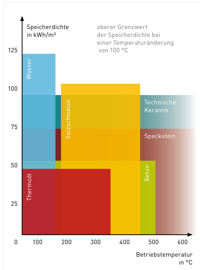
Abb. 3: Speichermedien für sensible Wärmespeicher
