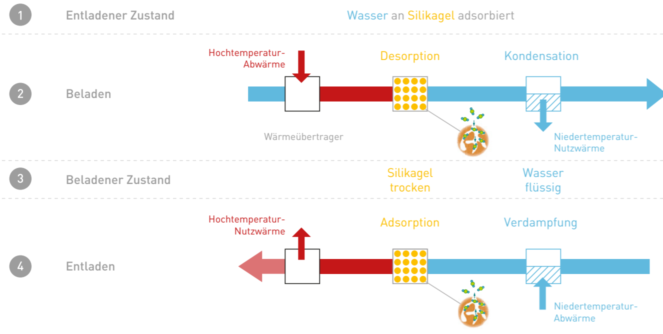
Abb. 36: Funktionsprinzip physisorptiver Speicher
