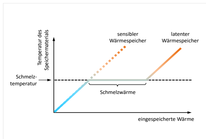
Abb. 32: Vergleich der Speicherkapazität eines sensiblen und eines latenten Wärmespeichers. Bei latenten Speichermedien findet der Wärmeübergang innerhalb kleinerer Temperaturdifferenzen statt. Zusätzlich zur Latentwärme wird auch die sensible Wärme des Speichermediums genutzt. Allerdings macht sie nur einen Bruchteil der nutzbaren Wärme aus.
