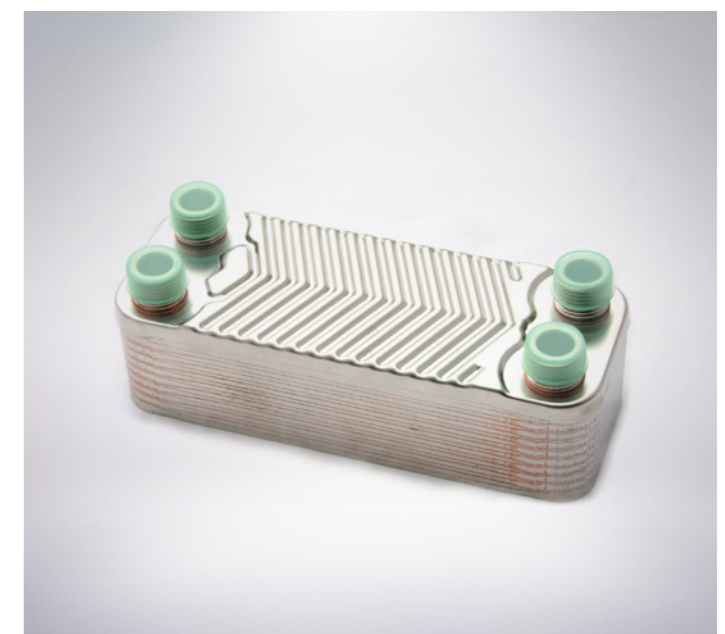
Plattenwärmeübertrager mit Stutzen für Kühl- und Heizmedium
