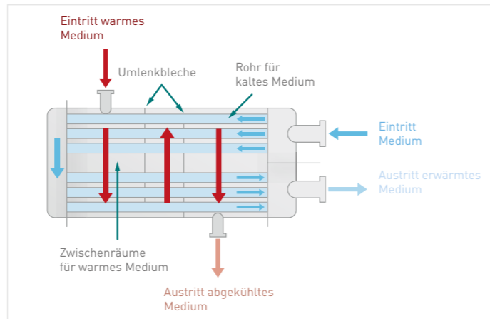
Abb. 9: Prinzip eines Rohrbündelwärmübertragers
