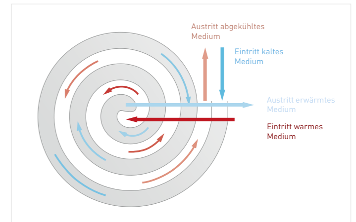
Abb. 19: Prinzip eines Spiralwärmeübertragers
