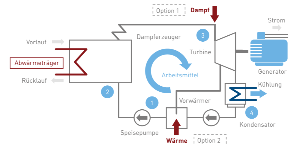
Abbildung x: Schaltbild eines Dampfkraftprozesses
