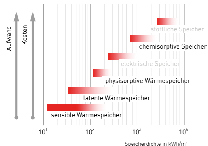
Abb. 24: Energiespeicherdichte verschiedener Arten von Wärmespeichern bei begrenzter Temperaturdifferenz. Zum Vergleich sind stoffliche Speicher (flüssige Brennstoffe) und elektrische Speicher (Batterien) angegeben.
