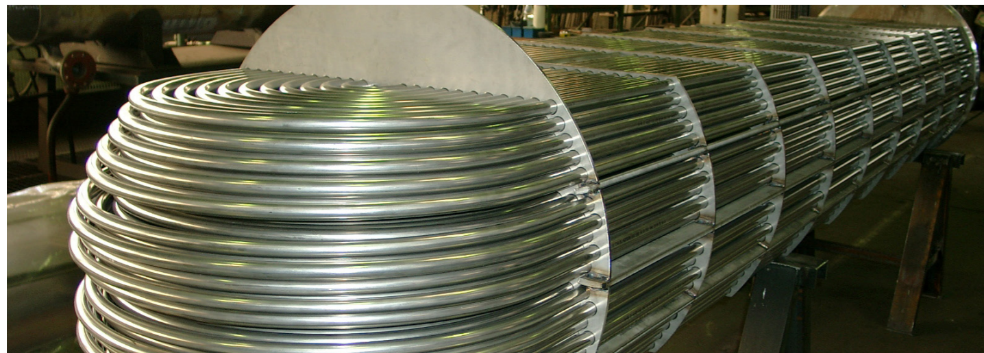
Rohrbündelwärmübertrager mit U-Rohren
