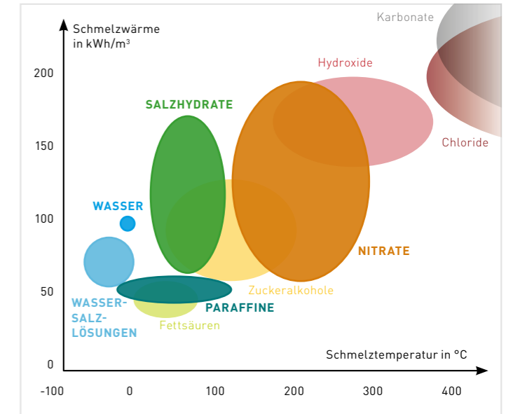
Abb. 31: Anwendungsbereich (Temperatur) und Speicherdichte (Schmelzwärme) unterschiedlicher Materialien für Latentwärmespeicher: Für Wasser, Wasser-Salz-Lösungen, Salzhydrate, Paraffine und Nitratsalze existieren kommerzielle Lösungen oder vielversprechende Pilotprojekte. Alle anderen Stoffe sind als Speichermedien in der Entwicklung. Mit Karbonaten und Chloriden ließen sich noch höhere Speicherdichten und Temperaturen (bis >700°C) erreichen.
