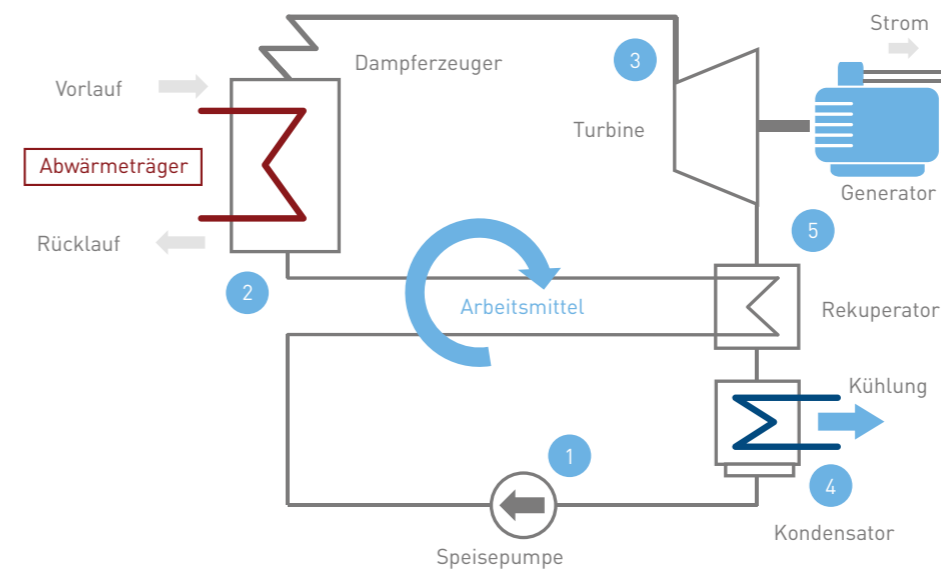
Abbildung 7: Schaltbild eines ORC-Prozesses
