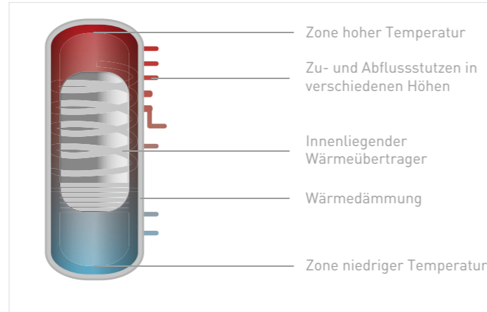
Abb. 4: Prinzipaufbau eines Warmwasserspeichers mit innenliegendem Wärmeübertrager
