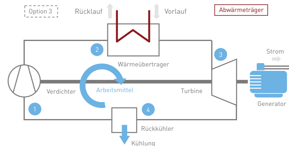
Abb. 9: Schaltbild eines Gasturbinenprozesses (geschlossen)
