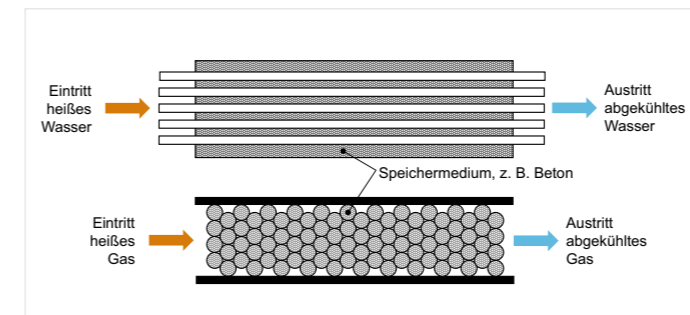
Abb. 6: Möglichkeiten des Aufbaus eines sensiblen Wärmespeichers mit festem Speichermedium. Dargestellt ist der Beladevorgang.
