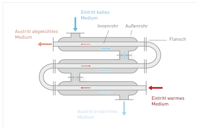
Abb. 15: Prinzipskizze eines Doppelrohrwärmeübertragers
