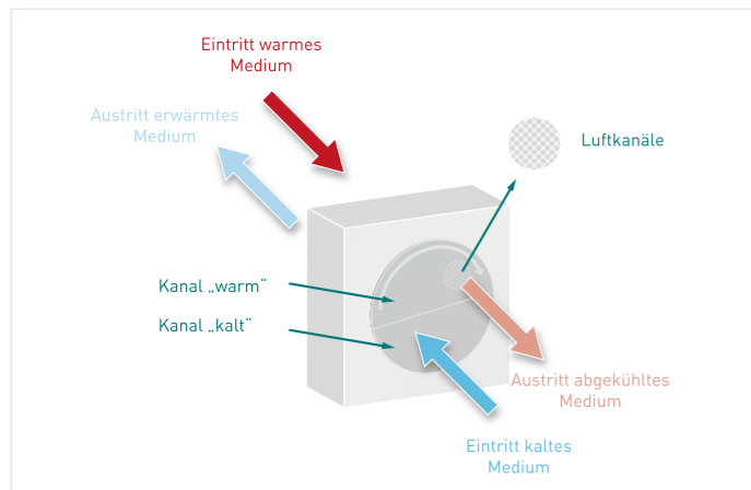
Abb. 23: Prinzip eines Rotationswärmeübertragers
