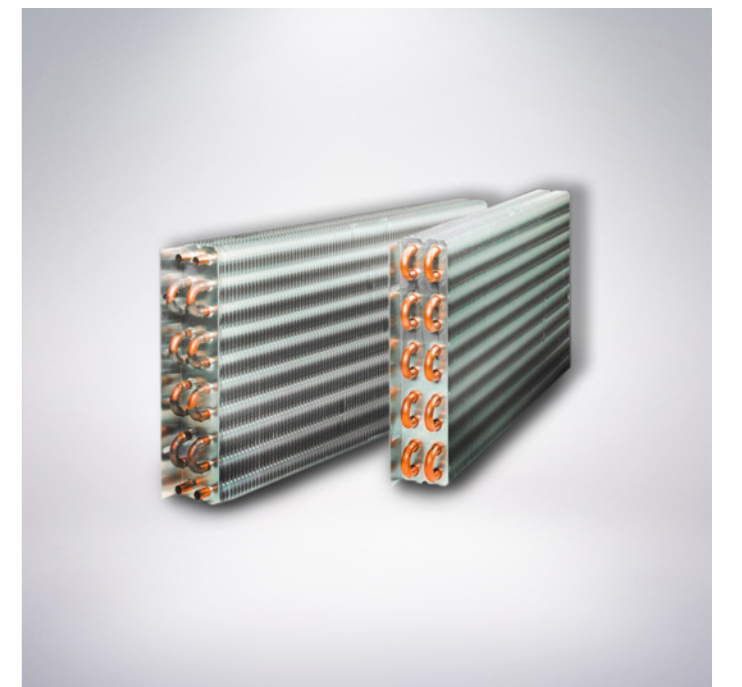
Lamellenwärmübertrager
