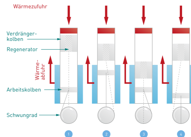
Abb. 11: Prinzip des Stirlingmotors
